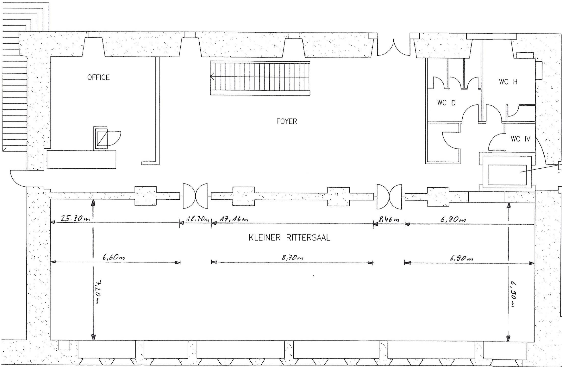
Kleiner Rittersaal Masstab 1:100
