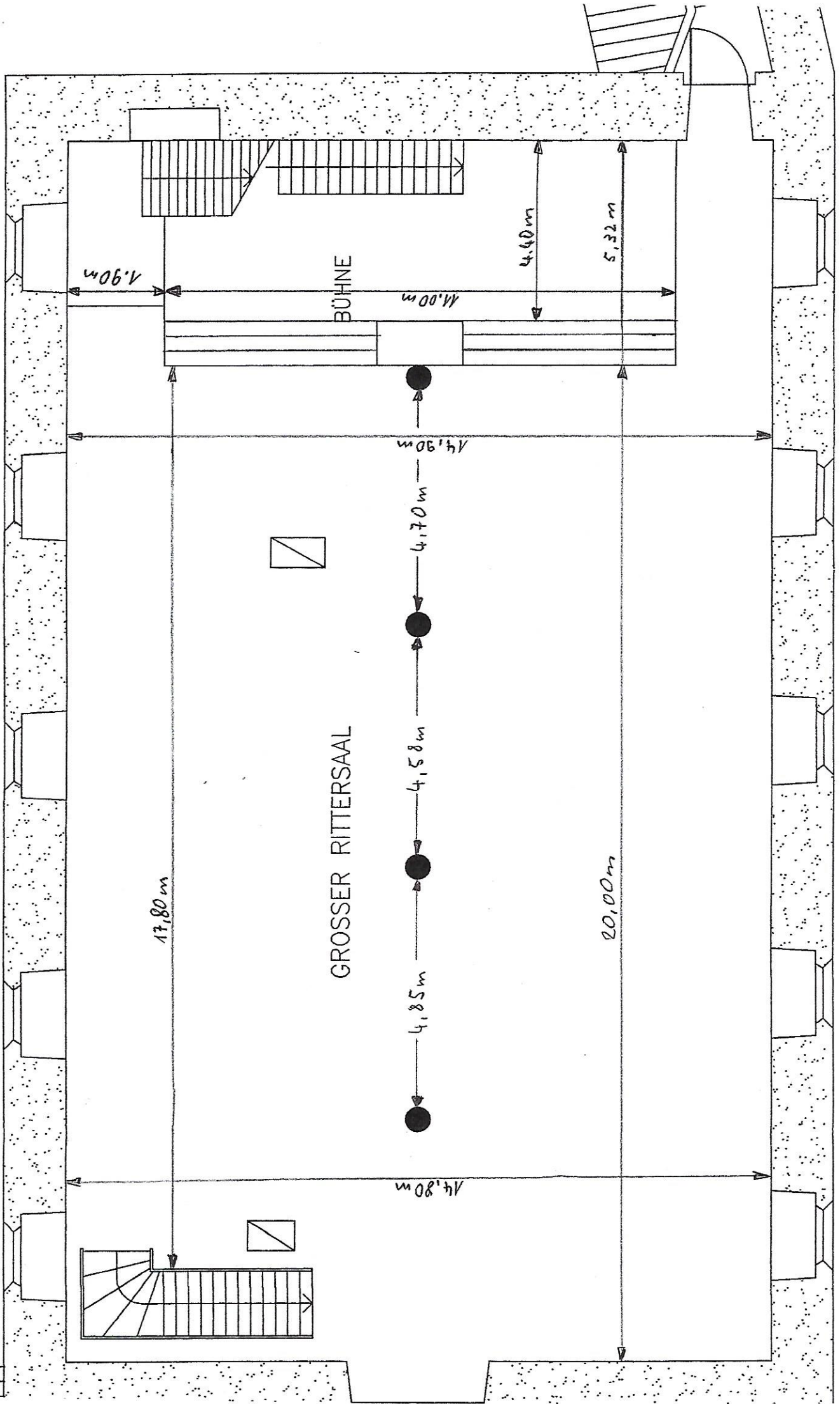
Grosser Rittersaal Masstab 1:100
